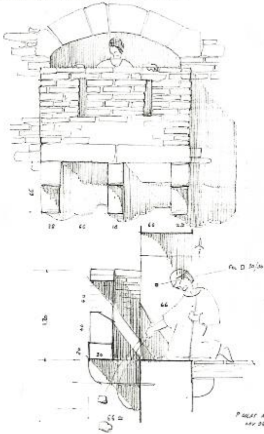
AIRE SUR L'ADOUR - CATHÉDRALE - RESTAURATION DE L'ÉCHAUGUETTE NORD DU CLOCHER.
